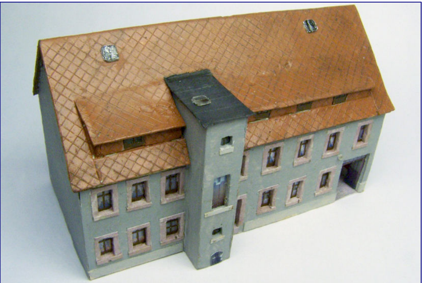
Die Nachbildung des Blechdaches (Bild oben) geschieht mit einer Acrylhaut, die in einer selbstgebauten Form erstellt wird. Sie legt sich auch fugenlos über die Dachgauben (Bild unten). Schwarze Papierstreifen, überlappend aufgelegt, bilden die Teerpappe auf dem Klo- und Zwerghausdach nach.
