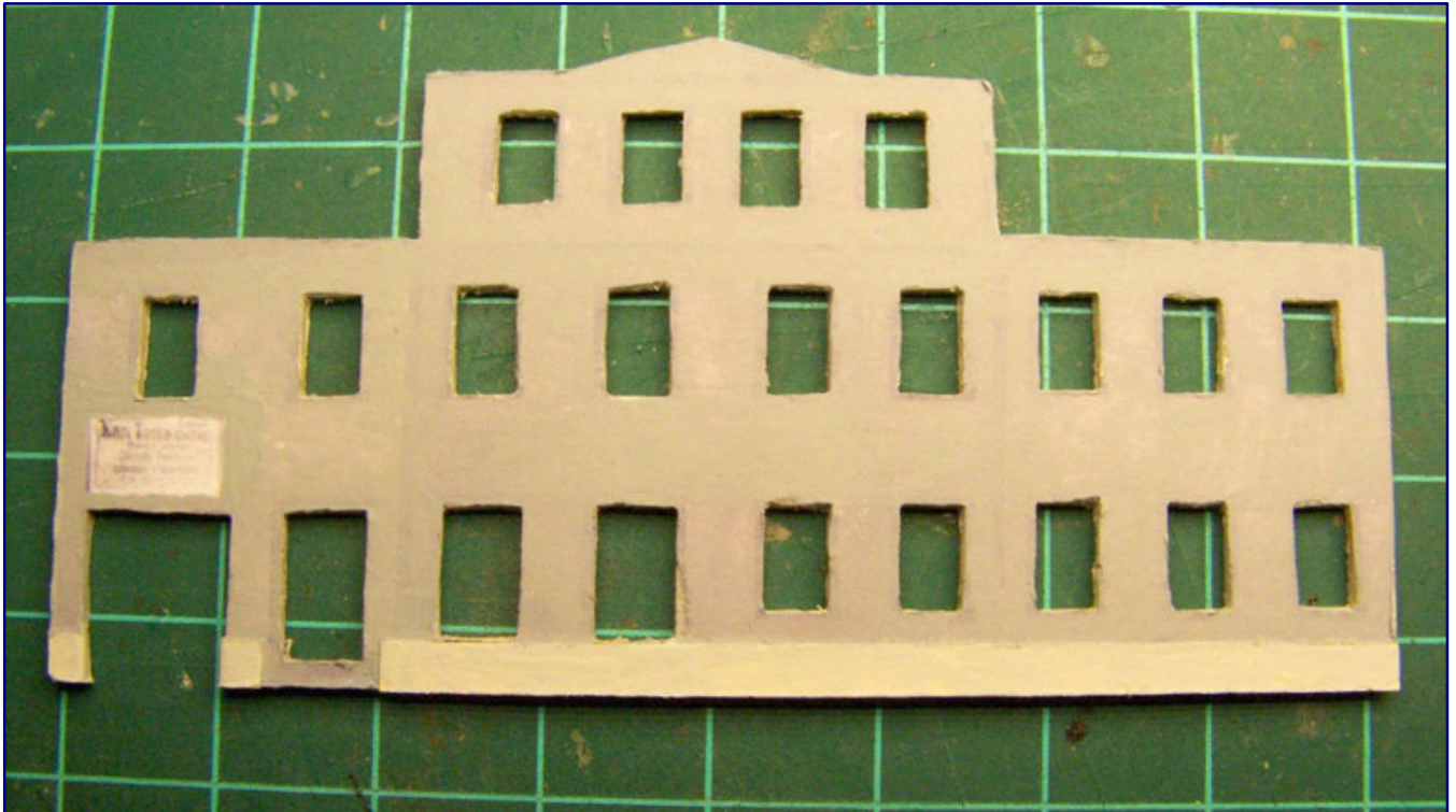
Nach dem Aussägen mit einem feinen Laubsägeblatt und Nacharbeiten mit der Nadelfeile wird der Tapetenkleber wieder gelöst und die Druckvorlage abgezogen. Die Hauswand ist nun bereit für ihren ersten Anstrich.
