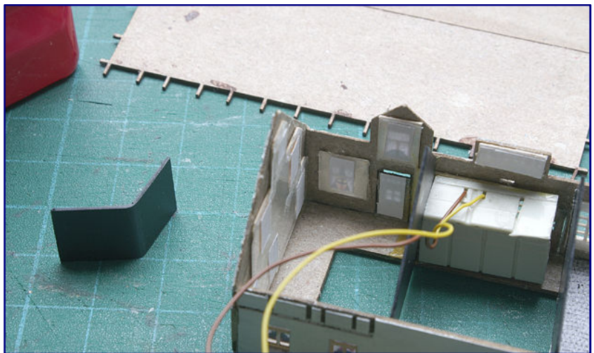
Aus schwarzen Evergreen-Bauplatten (Vertrieb über Faller) schneiden wir uns zwei Giebelwände zur Querversteifung (Bild oben). Zusammen mit den Teilen aus der Viessmann-Etagenbeleuchtung und dessen LED-Aufsatz werden sie auch Bestandteil des Lichtkastens (Bild unten). Da wir die Position einer Giebelwand gegenüber dem ursprünglichen Plan verändert haben, brauchen wir zusätzlich noch ein weiteres Stück schwarzen Polystyrols, um das Licht vollständig abzusichern.
