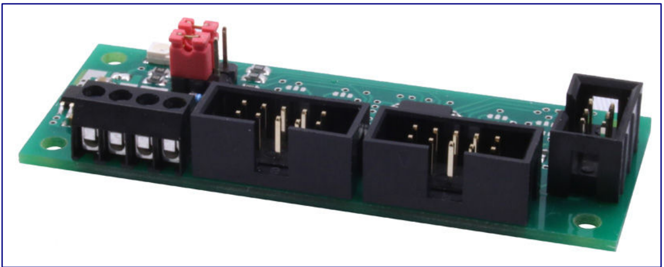
Der serielle Schalt-Bus als Sende-Modul (Art.-Nr. SSB64-S). Foto: Heißwolf Modellbahnzubehör.
