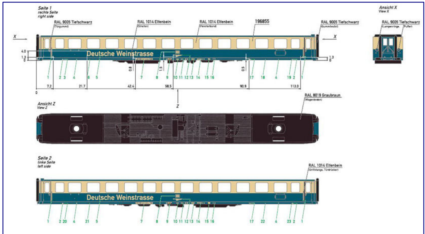
Entwurf für die Gestaltung des Laubenwagens WGM 824.4 „Deutsche Weinstraße“ (Art.-Nr. 98172), der vom 1zu220-Shop bei Märklin als Exklusiv-Modell beauftragt wurde. Abbildung: Märklin / 1zu220-Shop
