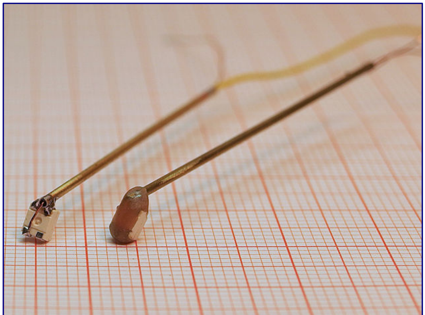
Bild oben: Das Anlöten der LED an den Mast wird leichter und gelingt in gleichen Winkeln, wenn eine geeignete Haltevorrichtung gebaut und genutzt wird.
