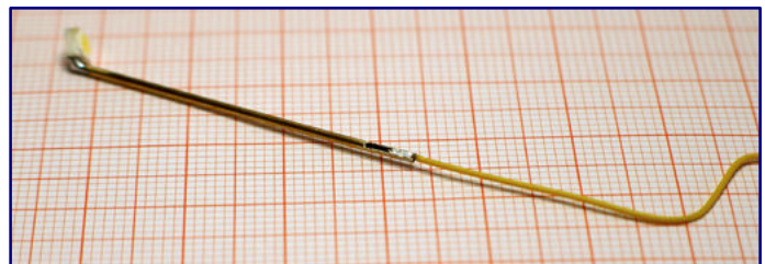
An die Abflachung wird das Kabel angelötet, um die elektrische Versorgung der Leuchtdiode zu sichern.
