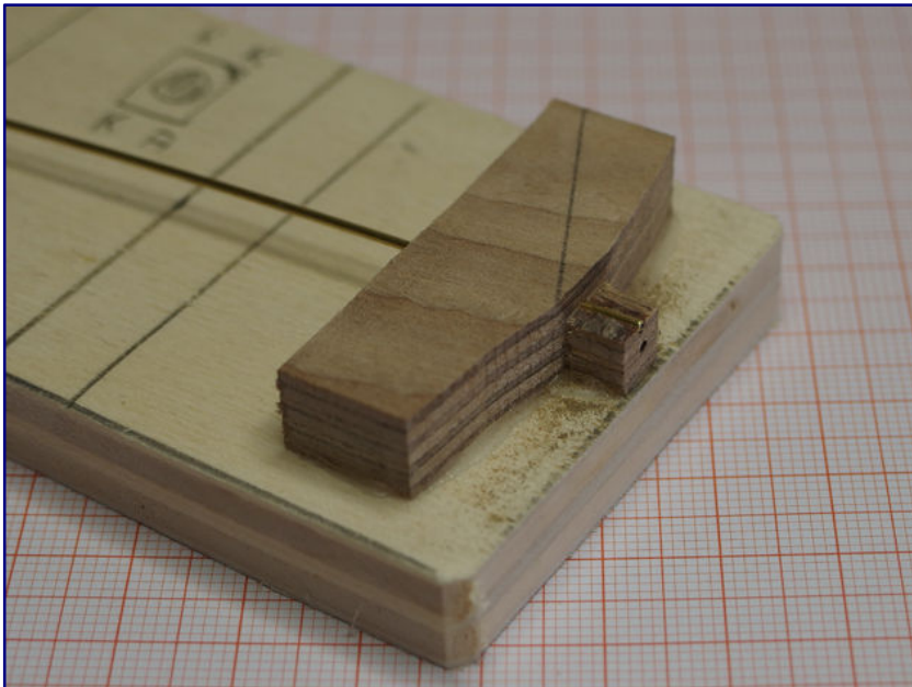
Mittels dieser Hilfsvorrichtung wird das Rohr problemlos und in korrekter Stärke abgeflacht.
