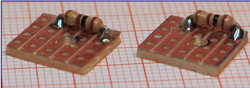
Eine einfache wie auch geeignete Anschlussplatine für die selbstgebauten Laternen könnte so wie auf diesem Bild aussehen.
