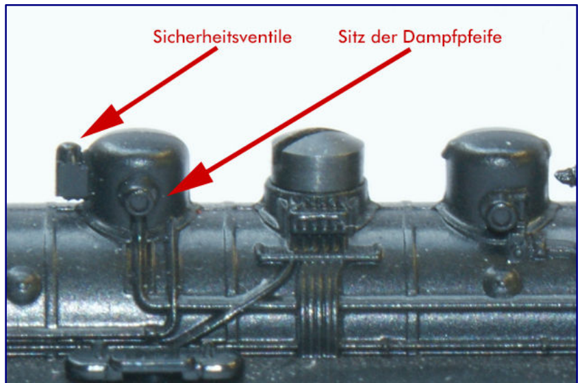
Am hinteren Ende des dritten Doms ist nur die Nachbildung von einem statt zwei Sicherheitsventilen erkennbar – und das wie auch die Handräder der Dampfentnahmeventile nur in stark vereinfachter Form. Die Dampfpeife - Pflichtausstattung jeder Dampflok - fehlt völlig. Sie sollte weit vorne auf der rechten Seite desselben Doms sitzen. Hier hätte Märklin Anschauungsunterricht am eigenen H0-Modell gleicher Betriebsnummer nehmen können.
