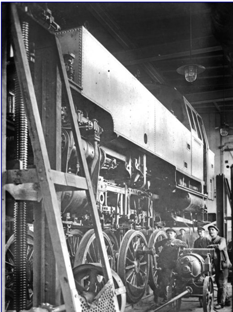
Diese Aufnahme zeigt den Bau der 64 214 im Jahre 1928 in der Lokomotivfabrik Hagans. Sie war die vorletzte dort gefertigte Lokomotive, im gleichen Jahr endete die Lokproduktion. Foto: Slg. Johannes Glöckner, Archiv Eisenbahnstiftung
