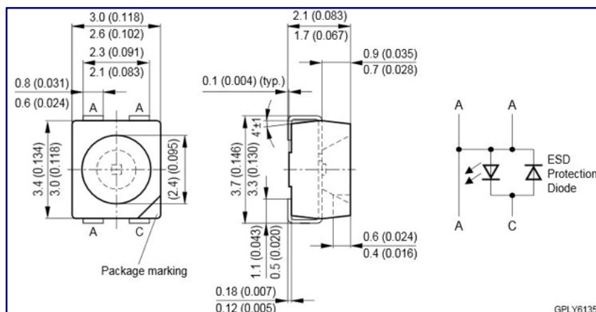
Auszug aus dem Osram-Datenblatt: links ein Blick auf die Leuchtseite der LED. Abbildung: Osram
