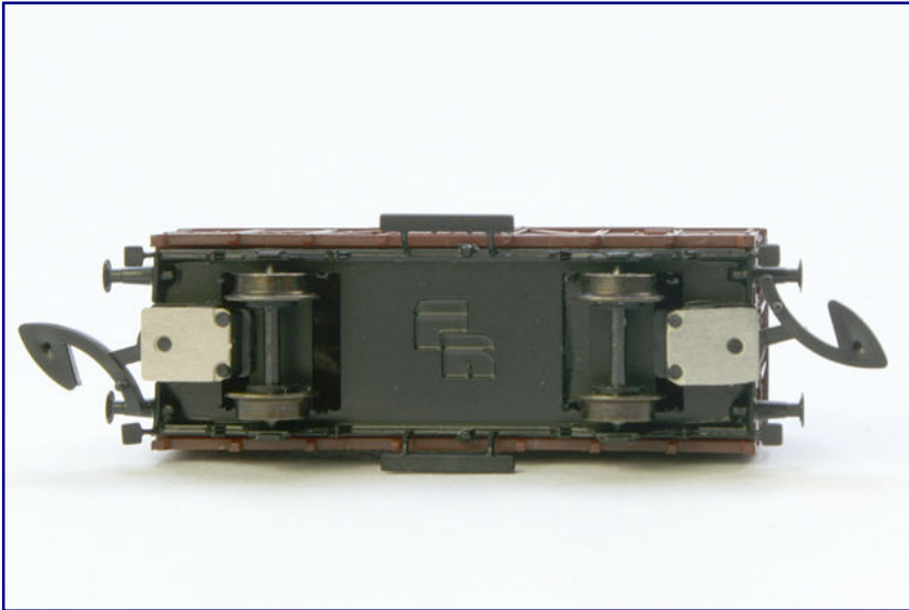
Ein Blick auf den Unterboden zeigt neben den Achsen mit Spitzenlagerung, den Kupplungen mit Schächten und am Fahrwerk sitzenden Trittblechen keine weiteren Details am Wagenboden.
