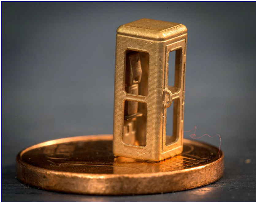
Eine Demonstration des Könnens: Märklin zeigte die Möglichkeiten des Messingfeingusses unter Einsatz des 3D-Drucks und verlorener Formen am Beispiel einer Telefonzelle für die Spurweite Z.
